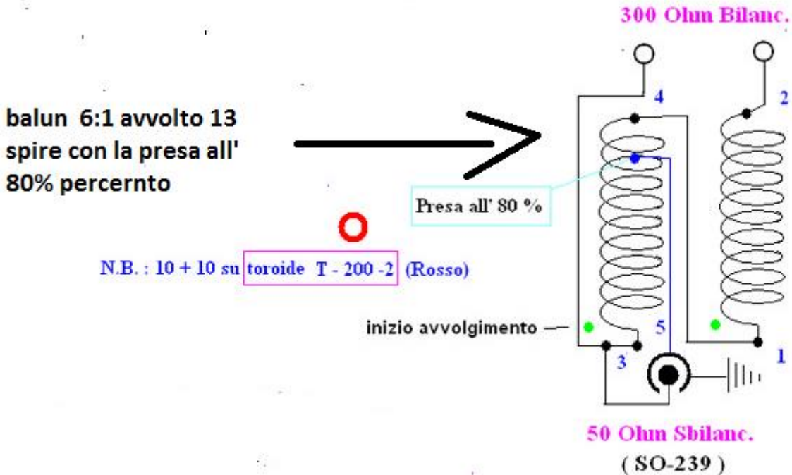
Fig 3: schema balun 6:1
